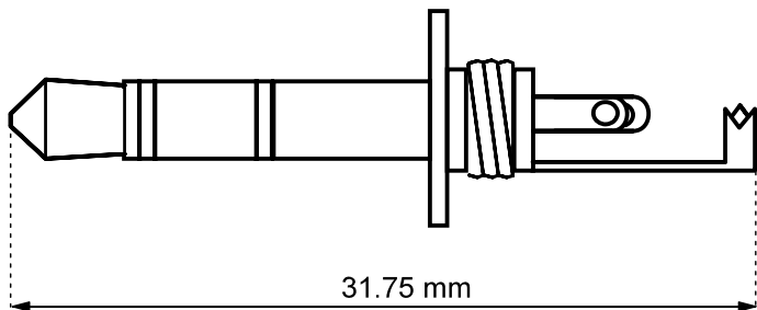
Stecker plug
